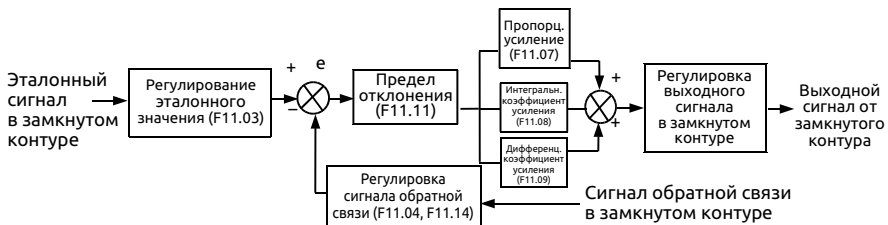
Рис. 7-37 Схема принципа работы ПИД-регулятора
