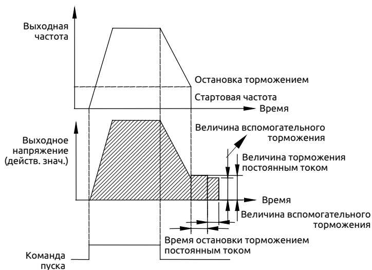
Рис. 7-5 Торможение до останова + торможение постоянным током
